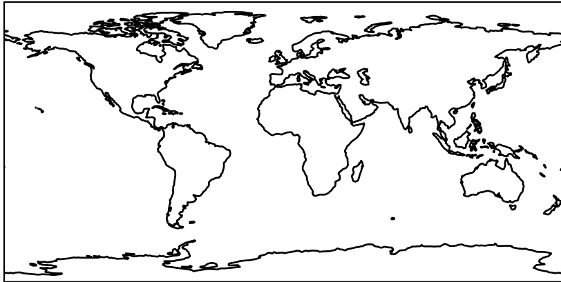
gchp.14.5.0-rc.0 (Ref) c24
