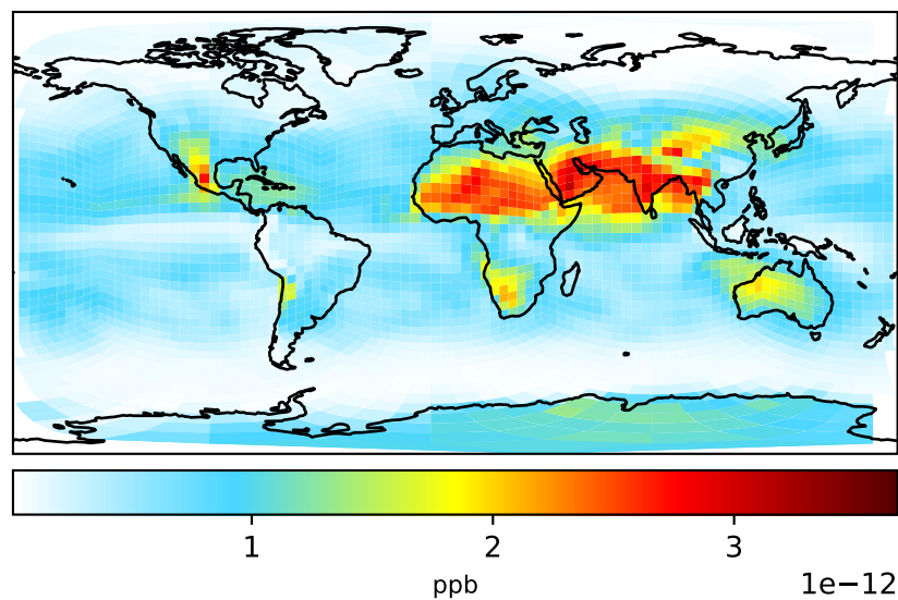
gchp.14.7.0-rc.0-LuoWD (Dev) c24
