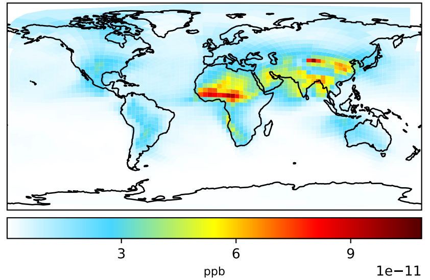
gchp.14.7.0-rc.0-LuoWD (Dev) c24
